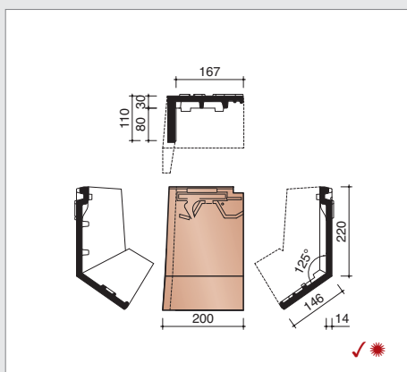
MVBD7280 Linker gevelknikpan op maat (verlijmd)
