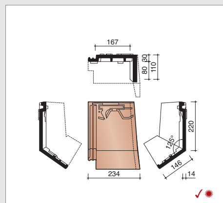
MVBD7290 Rechter gevelknikpan op maat (verlijmd)
