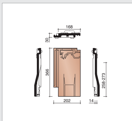
MVBD8640 Ventilatiepan met rooster in kunststof 10 cm 2
