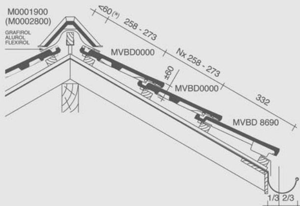
Dwarsdoorsnede dak ter hoogte van hoekige vorst Vauban
