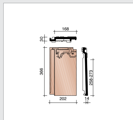
MVBD8690 5,9 stuks/lm Dakgootventilatiepan
