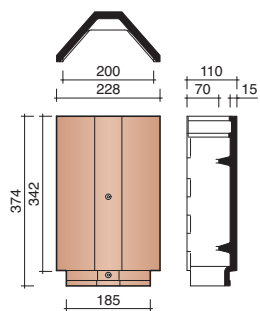
M0002800 3 stuks/lm Hoekige vorst - noordboom Actua
