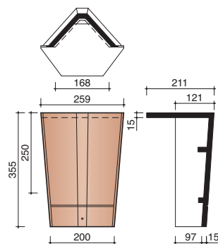
M0001910 Hoekige beginvorst Vauban
