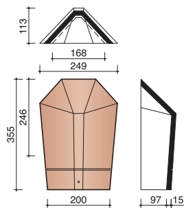
M0001960 Hoekige beginnoordboom Vauban
