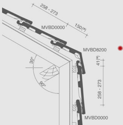
Lengtedoorsnede dak ter hoogte van haakvorst
