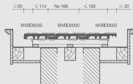
Dwarsdoorsnede dak ter hoogte van pan zonder zijsluiting
