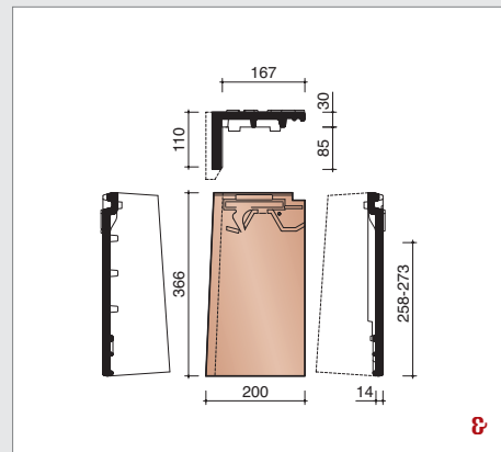
MVBD7080 1,9 stuks/lm Linker gevelpan
