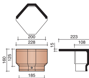
M0002810 Hoekige beginvorst Actua
