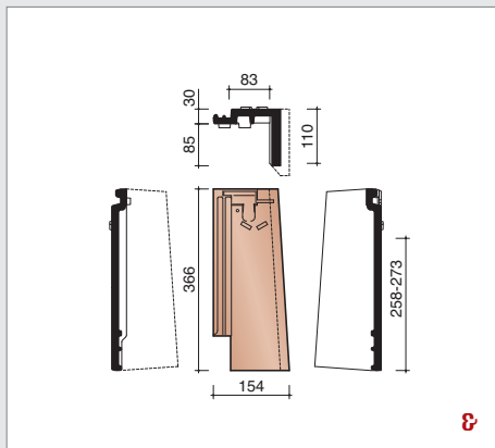
MVBD7030 1,9 stuks/lm Halve rechter gevelpan
