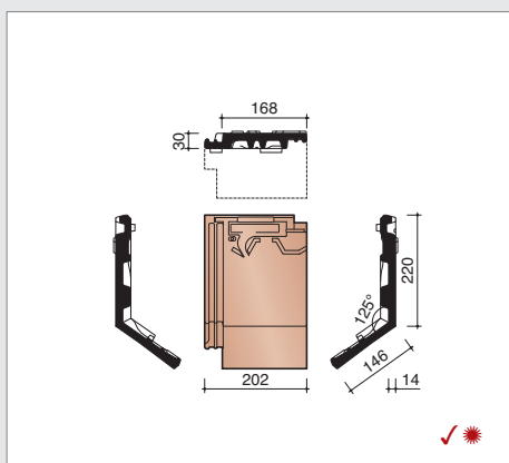
MVBD8200 5,9 stuks/lm Knikpan op maat (verlijmd)
