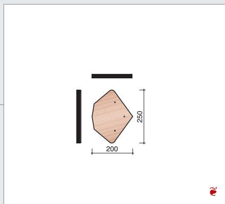
M0002240 Koplaat voor universele haakvorst
