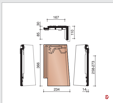
MVBD7090 1,9 stuks/lm Rechter gevelpan
