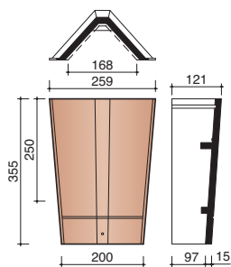
M0001900 4 stuks/lm Hoekige vorst - noordboom Vauban
