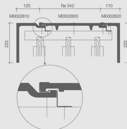
Dwarsdoorsnede dak ter hoogte van hoekige vorst Actua
