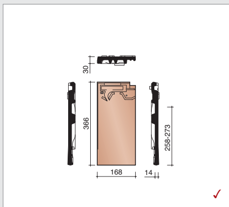
MVBD8050 1,9 stuks/lm Linker zijpan zonder sluiting
