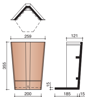
M0001920 Hoekige eindvorst Vauban
