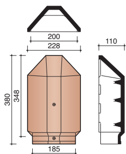
M0002860 Hoekige beginnoordboom Actua
