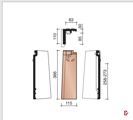
MVBD7020 1,9 stuks/lm Halve linker gevelpan
