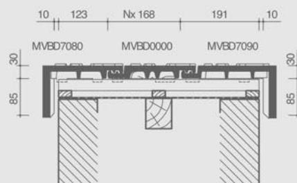
Dwarsdoorsnede dak ter hoogte van gevelpannen
