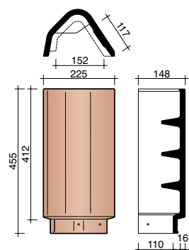
M0002200 2,4 stuks/lm Universele haakvorst
