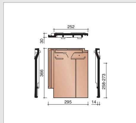
MVBD8080 1,9 stuks/lm Rechter anderhalve zijpan
