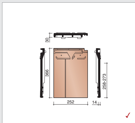
MVBD8070 1,9 stuks/lm Linker anderhalve zijpan zonder sluiting
