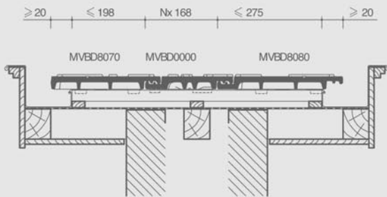
Dwarsdoorsnede dak ter hoogte van anderhalve pan zonder zijsluiting
