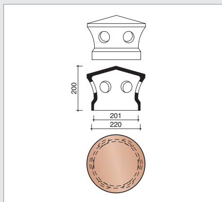
M0008780 Kapje voor kokerpan Ø 150 mm
